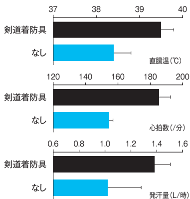
図 23 剣道着と防具を着用すると、直腸温、心拍数、発汗量がいずれも顕著に高くなります。同じ運動をしても(60分間)、剣道着・防具の着用が大きな熱ストレスになっていることがわかります。(P99,2001)
